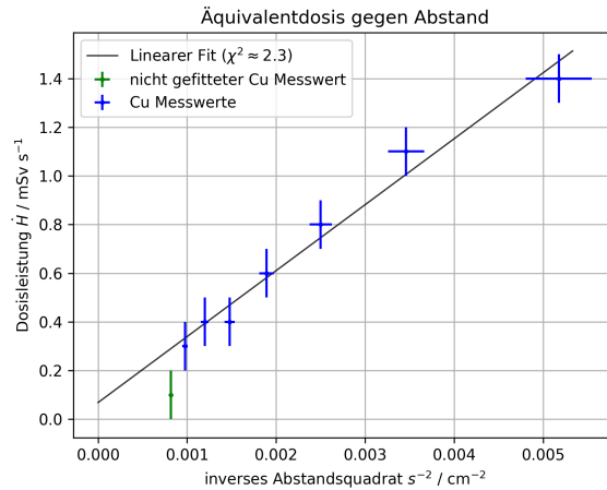
Abbildung 19: Linearer Fit der Äquivalentdosis H über Integrationszeit \Delta t = 1 s gegen inverses Abstandsquadrat s^{-2} (Kupfer-Röhre, I = 0,1 mA, U = 35 kV)
