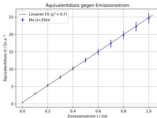
Abbildung 17: Äquivalentdosis H pro Jahr in Abhängigkeit des Emissionsstroms I (Molybdän-Röhre, U = 35 \text{ kV} )
