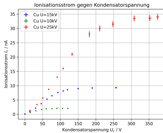
Abbildung 14: Ionisationsstrom I_C des Kondensators in Abhängigkeit der Kondensatorspannung U_C für drei verschiedene Röhrenspannungen (Kupfer-Röhre, I = 1 \text{ mA} )
