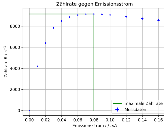
Abbildung 21: Zählrate R gegen Emissionsstrom I (Kupfer-Röhre, U = 35 \text{ kV} )
