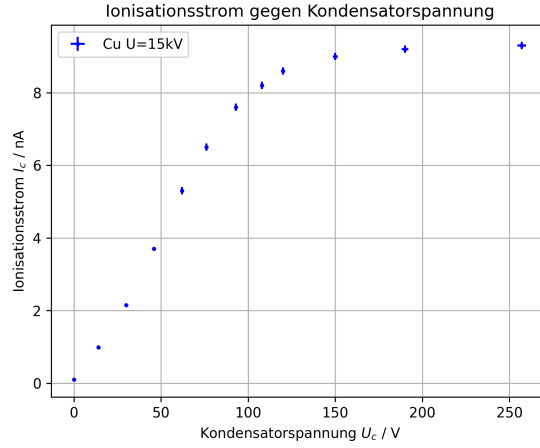
Abbildung 13: Ionisationsstrom I_C des Kondensators in Abhängigkeit der Kondensatorspannung U_C für Röhrenspannung U = 15 \text{ kV} (Kupfer-Röhre, I = 1 \text{ mA} )
