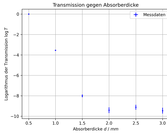
Abbildung 23: Logarithmus des Transmissionsgrads \log T gegen Absorberdicke d (Molybdän-Röhre, U = 35 \text{ kV} , mit Zirkoniumfilter)
