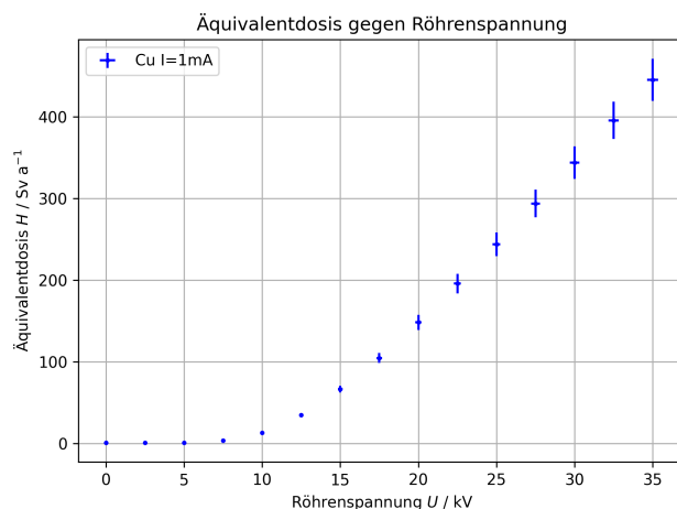
Abbildung 18: Äquivalentdosis H pro Jahr in Abhängigkeit der Röhrenspannung U (Kupfer-Röhre, I = 1 \text{ mA} )
