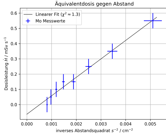
Abbildung 20: Linearer Fit der Äquivalentdosis H über Integrationszeit \Delta t = 2 s gegen inverses Abstandsquadrat s^{-2} (Molybdän-Röhre, I = 0,2 mA, U = 35 kV)
